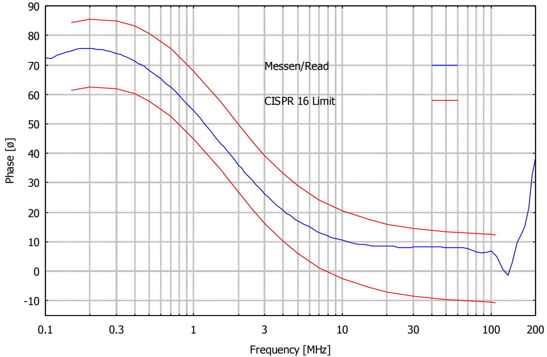
Phase an den Prüflingsklemmen (Spezialadapter erforderlich), N mit 50 \Omega Abschluss, Speiseklemmen offen Phase at EuT-terminals (adapter required), N-port is terminated with 50 Ohm, mains terminals open
